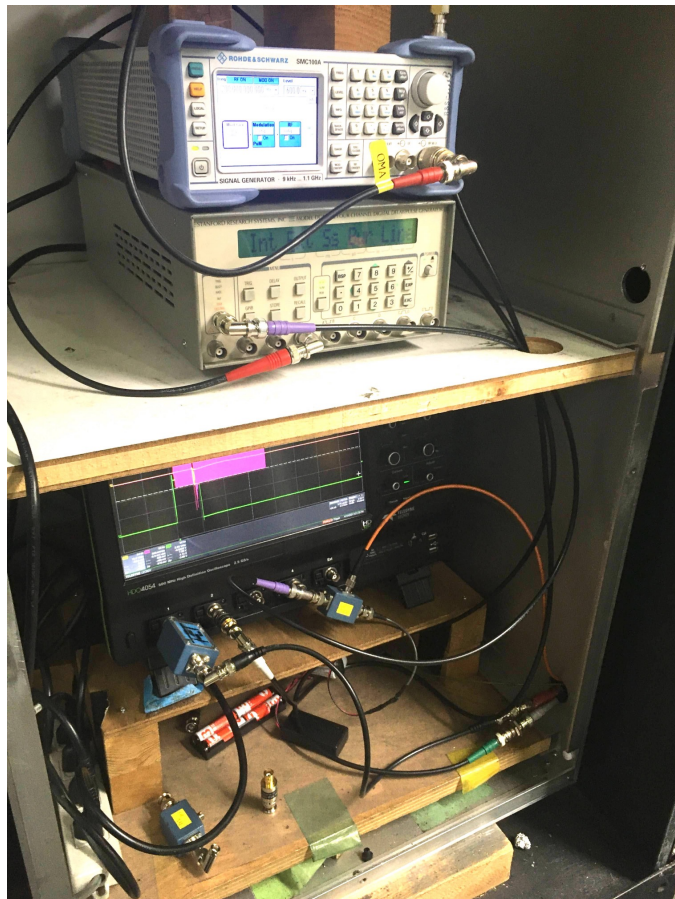
RF測定用のセットアップ
